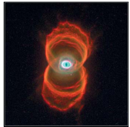
3. La jeune nébuleuse planétaire du Sablier (Hourglass Nebula, MyCn18) située dans la constellation de la Mouche à environ 8.000 années-lumière de nous. (© NASA/ESA)
